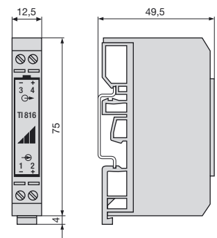
Fig. 10. SINEAX TI 816 on top-hat rail EN 50 022 - 35 x 7.5.
