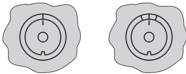
Fig. 5. Point mécanique de zéro à gauche: pour convertisseurs de mesure d'angle de rotation avec étendues 0 à ... \pm\alpha , à droite: pour convertisseurs angulaires avec caractéristique V.
