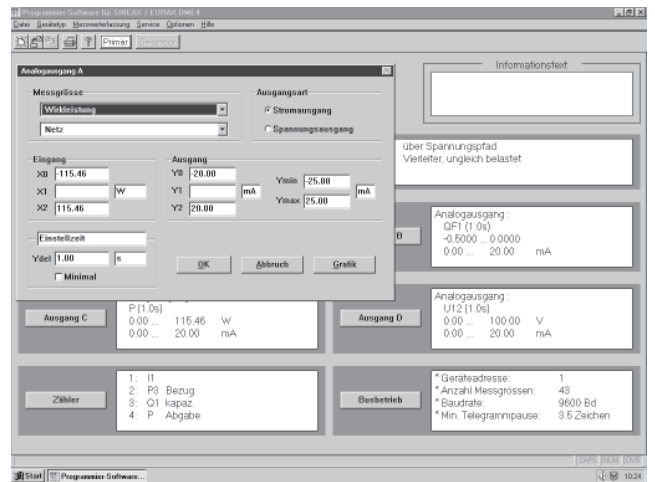
Bild 13. Programmierung der Ausgangs-Messgrössen.
