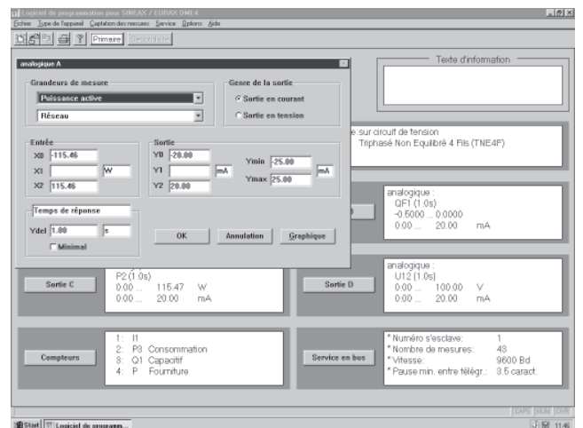
Fig. 13. Programmation des grandeurs de sortie.
