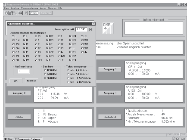
Bild 14. Auswahl der Busmessgrössen.
