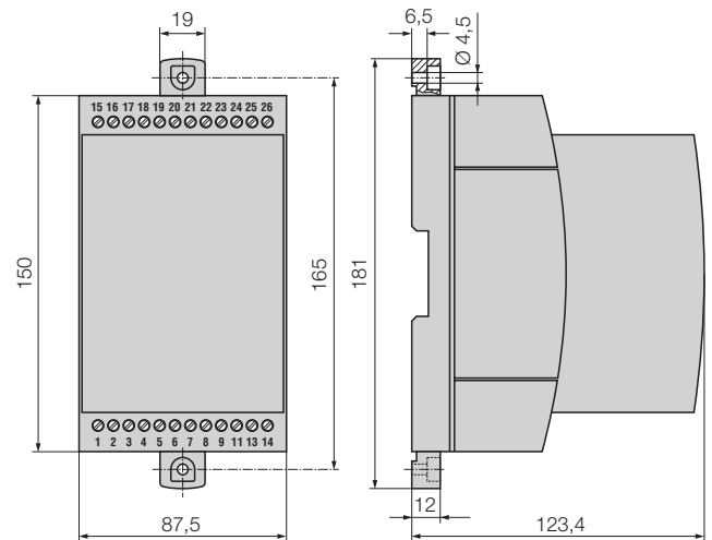
Bild 12. SINEAX DME im Gehäuse T24 mit herausgezogenen Laschen für direkte Wandmontage.
