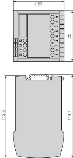
Bild 2. Gehäuse P19/70 auf Hutschiene (65 x 15 mm oder 35 x 7,5 mm, nach EN 50 022) aufgeschluppt.
