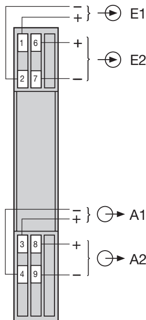
Bild 8. Typ 807-122..., Ex-Ausführung (Eingangssignale E1 und E2 «eigensicher»)
